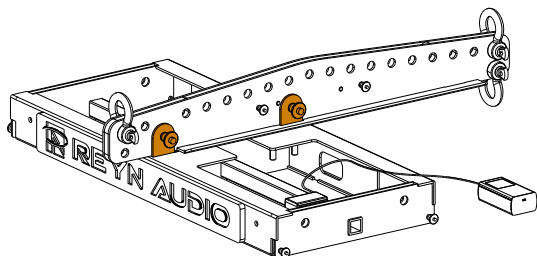
正常安装
