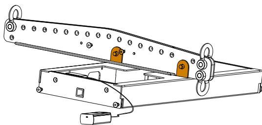
前移安装
